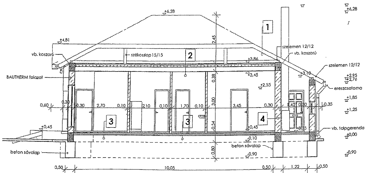
A/2 metszet m 1:100
