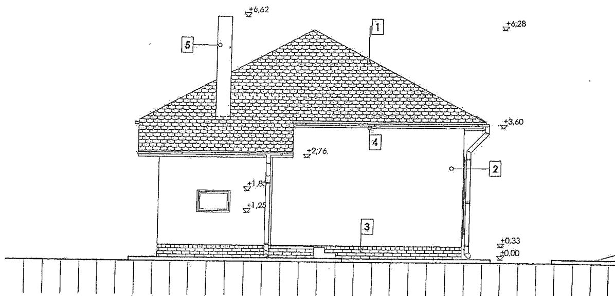
délnyugati homlokzat m 1:100
