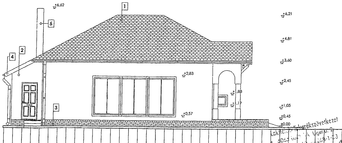
délkeleti homlokzat m 1:100
