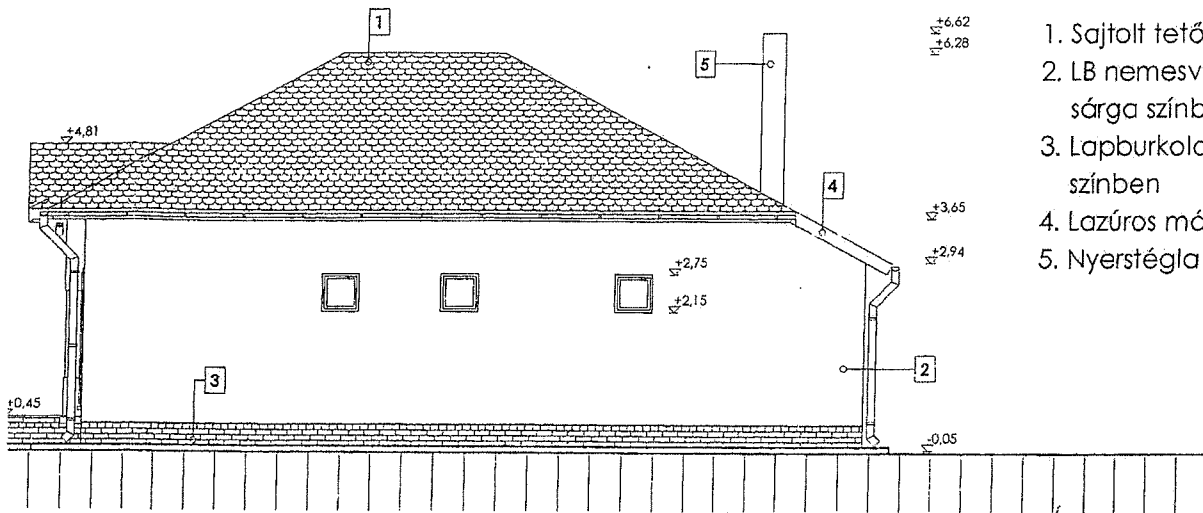
északnyugati homlokzat m 1:100
