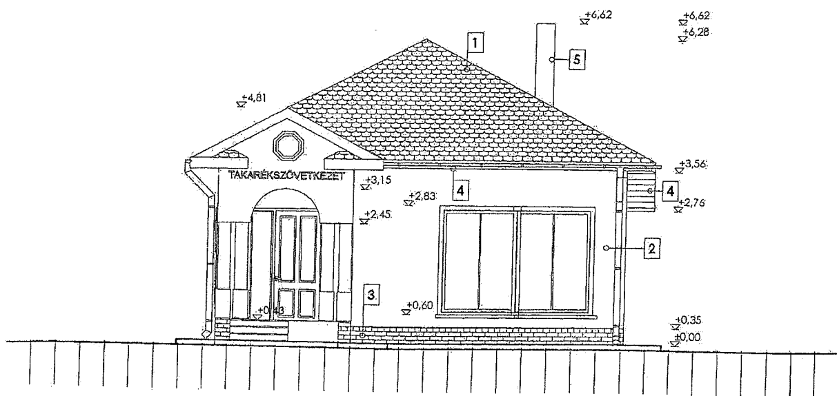
északkeleti homlokzat m 1:100
